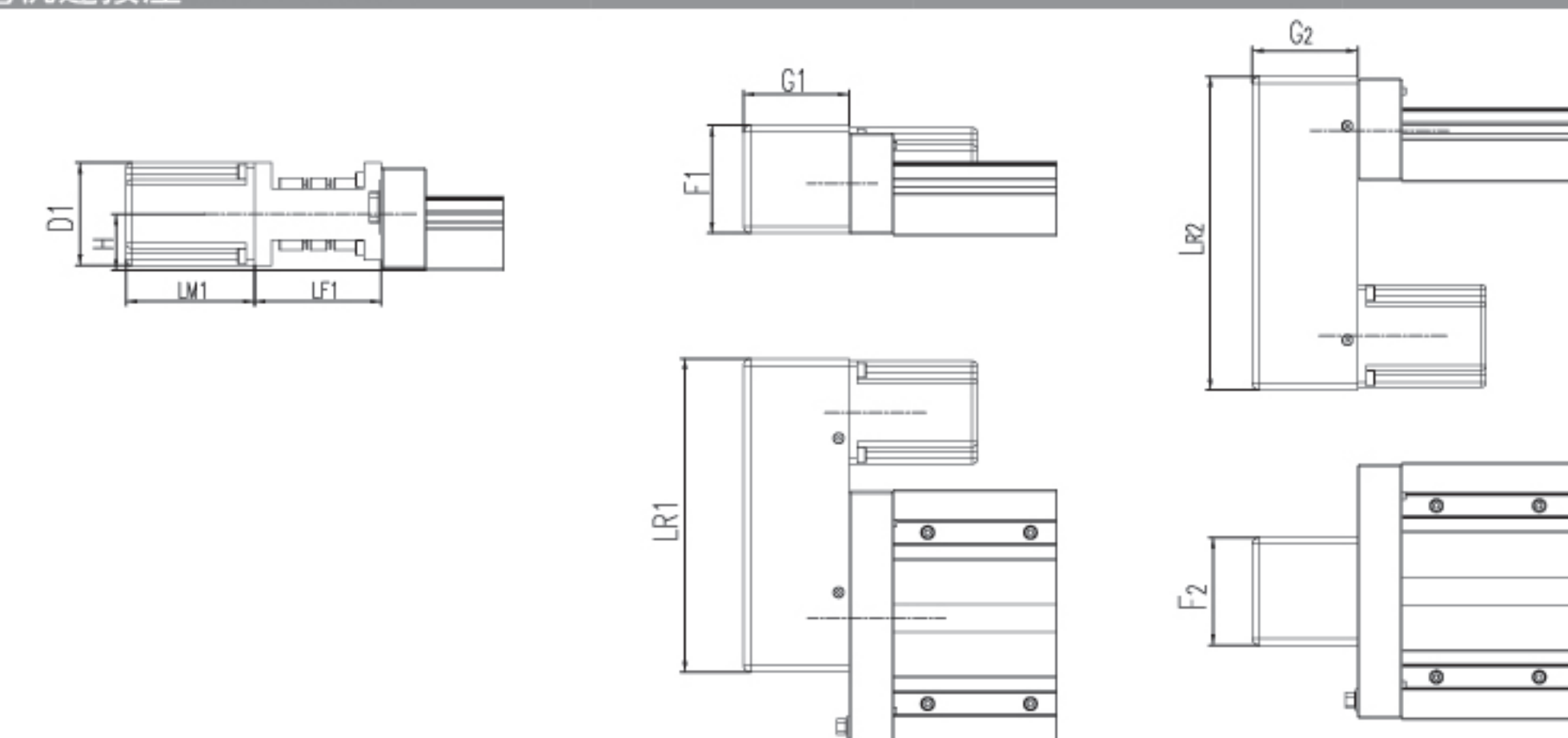
TSY320电机连接座 Motor socket
